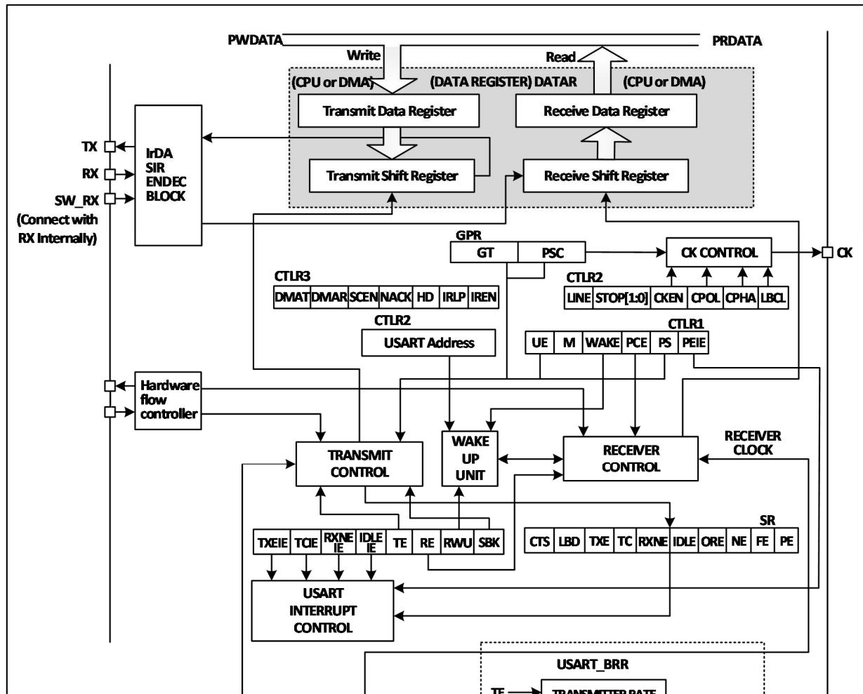
图 18-1 通用同步/异步收发器的结构框图
