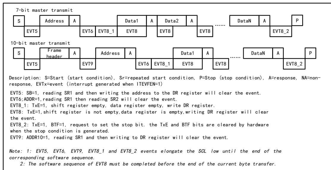
图 19-4 主发送器传送序列图
