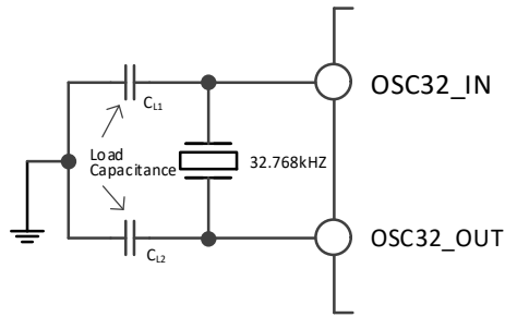
图 3-8 低速外部晶体电路
