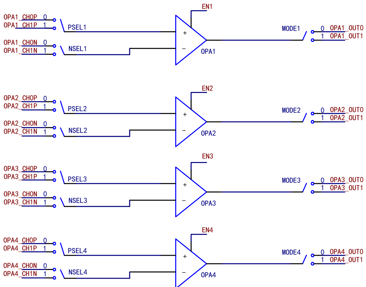
图 30-1 OPA 结构框图
