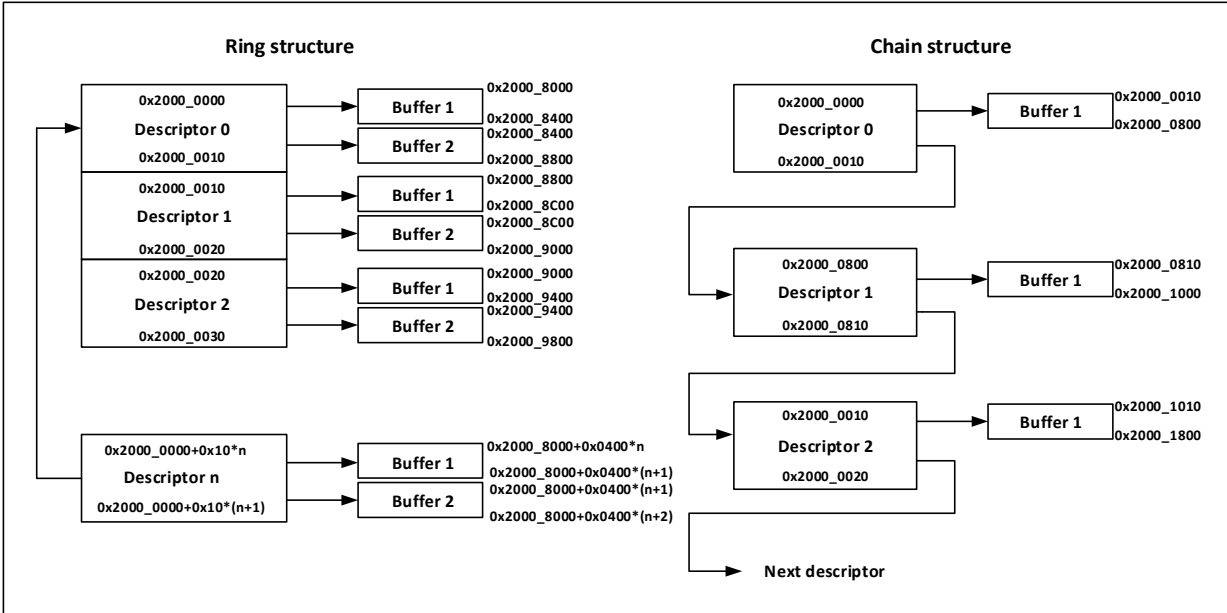
图 27-11 分别描述了环式结构和链表结构的一种缓冲区分配方案，供用户分配空间时参考。
