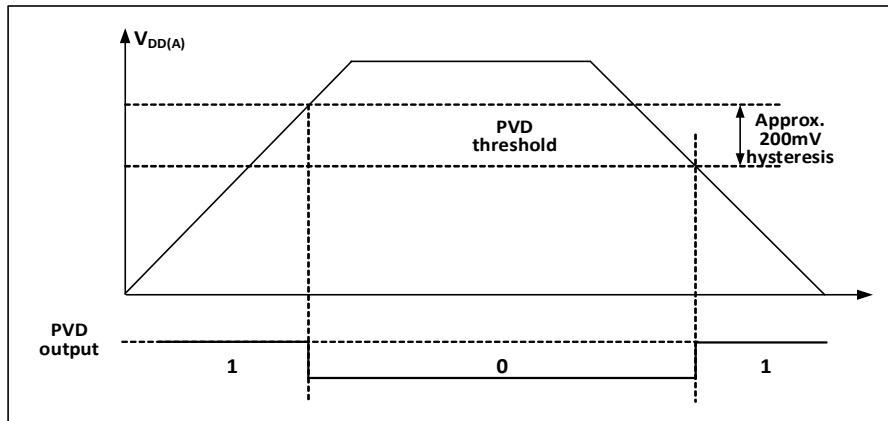
图 2-3 PVD 的工作示意图
