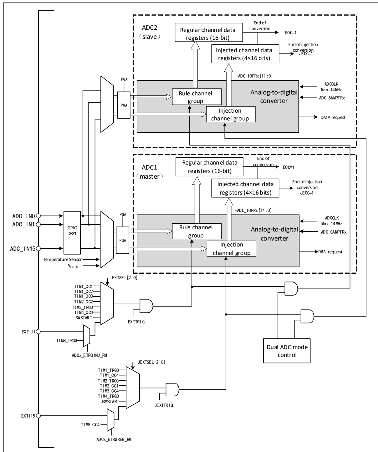
图 12-5 双 ADC 框图
