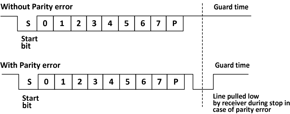
图 18-4 （未）发生奇偶校验错误示意图
