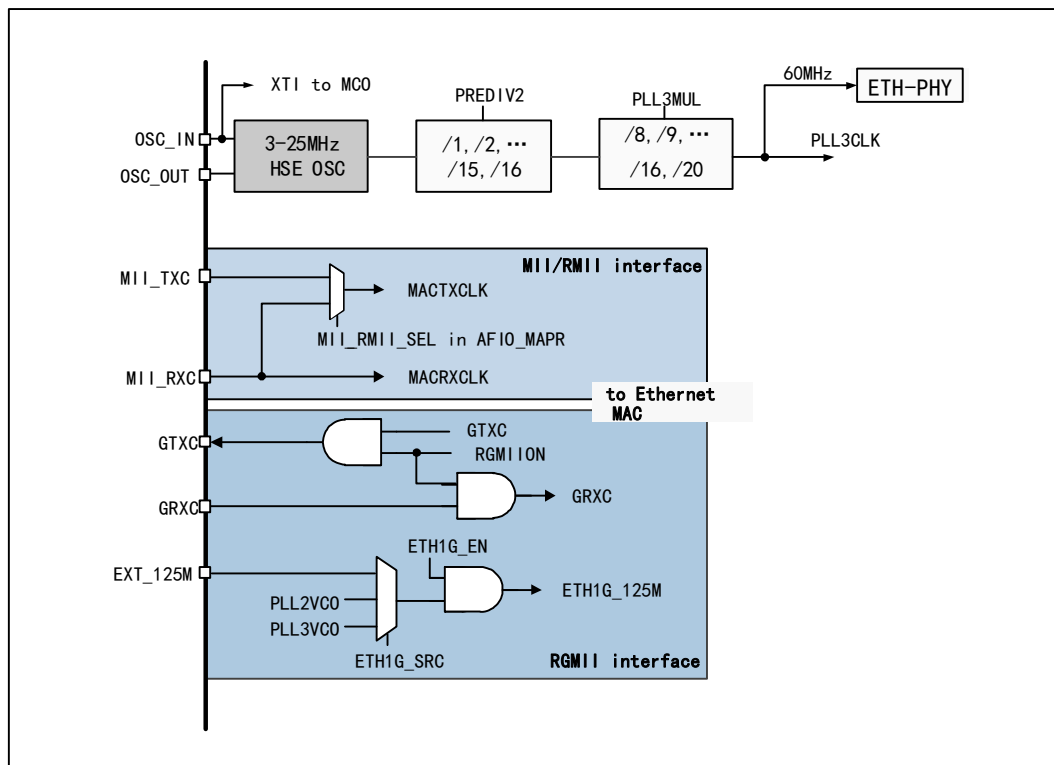
图 27-8 以太网外设时钟树
