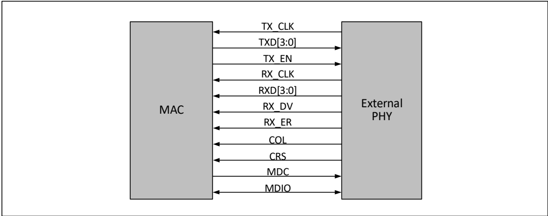
图 27-4 以太网收发器使用 MII 接口，MAC 和 PHY 如何接线
