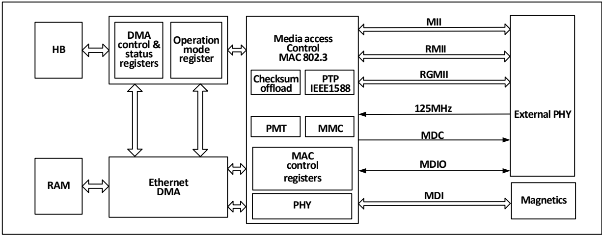
图 27-2 以太网收发器的结构框图
