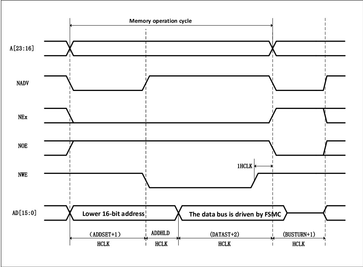
图 26-8 模式 B 写操作（复用）
