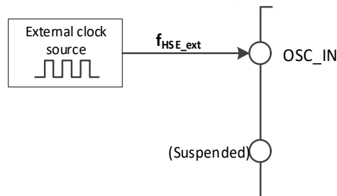
图 3-7 高速时钟源电路
